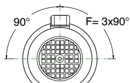
1LA5 56 - 80
