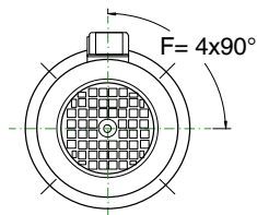
1LA5 90 - 160
